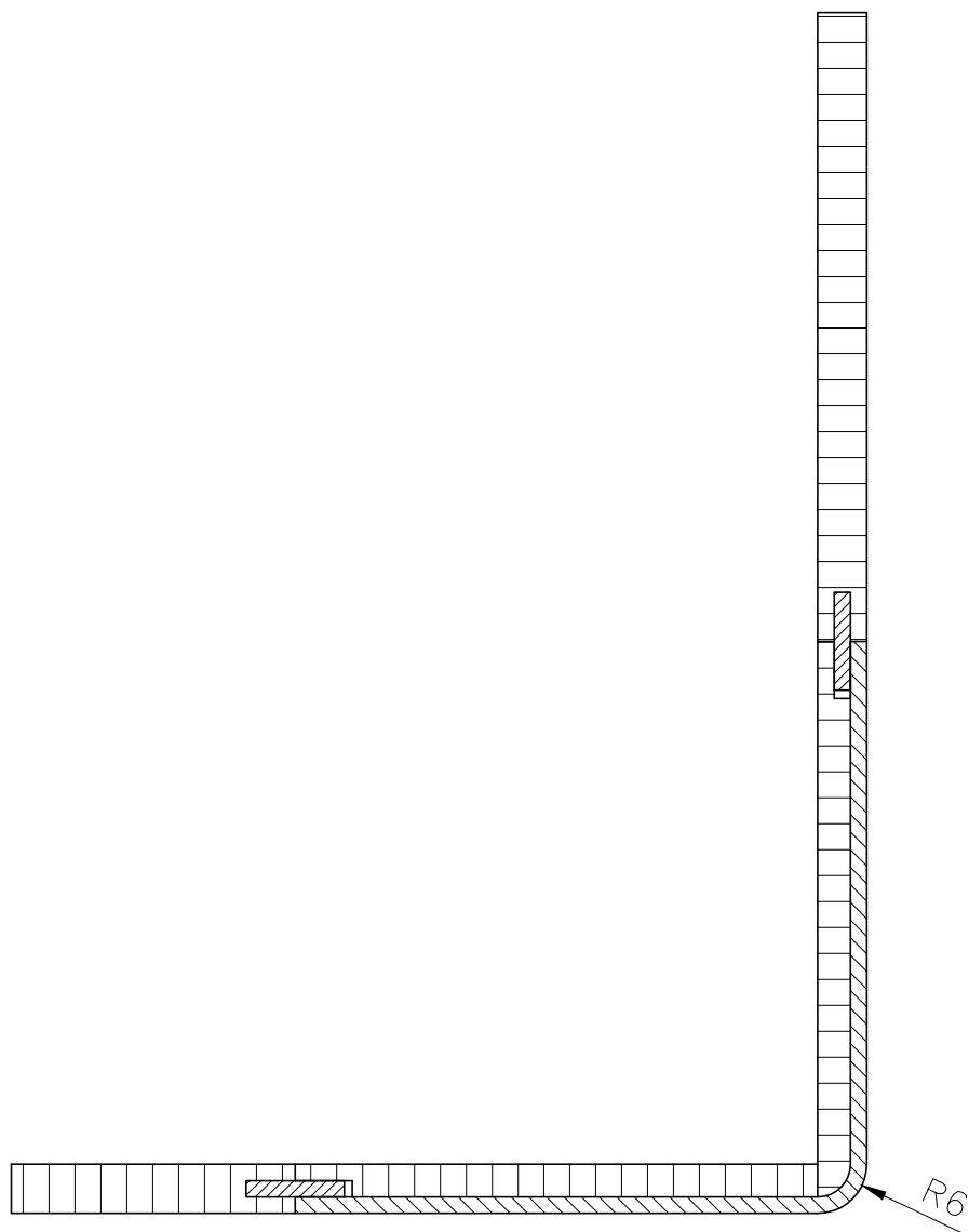
Edelstahlformteil
